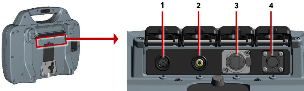
Fig. 3-4: Hoofdaansluitingspaneel
