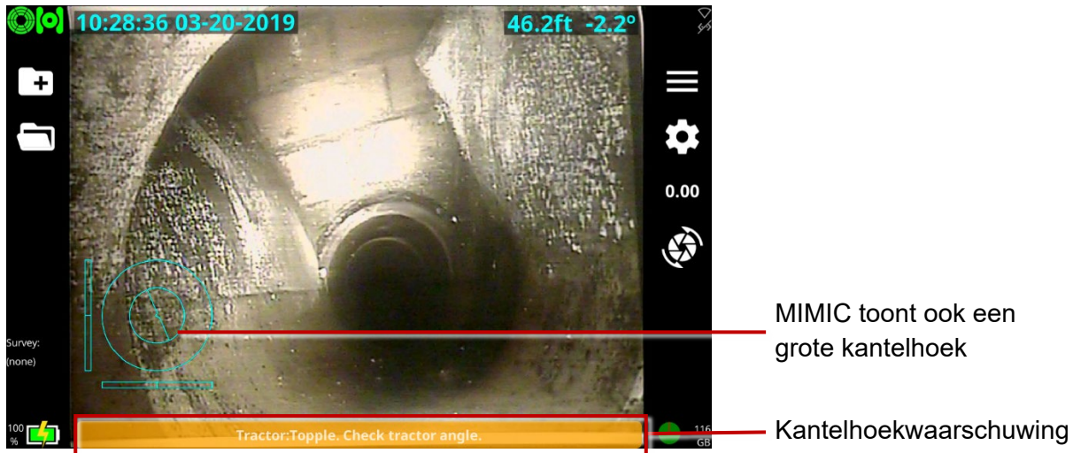
Fig. 6-14 Onderaan het scherm verschijnt de Kantelwaarschuwing. Merk op dat de MIMIC ook een grote kantelhoek weergeeft.
