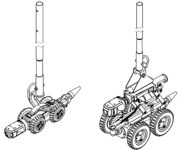
Fig. 4-18: Inzettool
