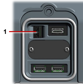
Fig. 5-1: Zekeringhouder (1) in het hulpaansluitingspaneel.
