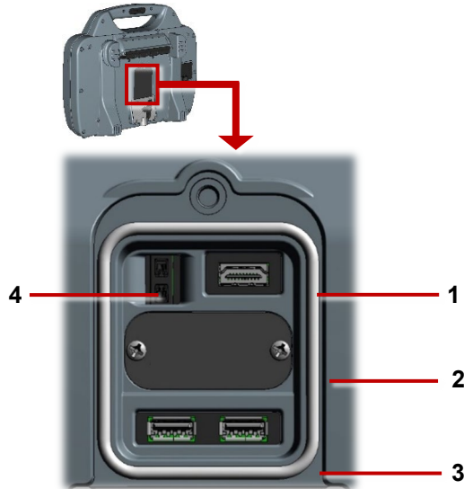
Fig. 3-5: Hulpaansluitingspaneel
