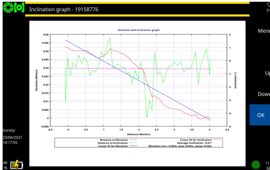
Fig. 6-27 Hellingsgrafiek.
