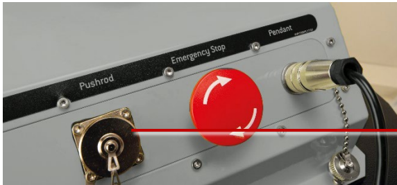
Fig. 4-22: Bus voor de verbinding van de 550c-duwkabel
