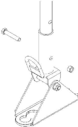
Fig. 6-6 Montage lifthouder
