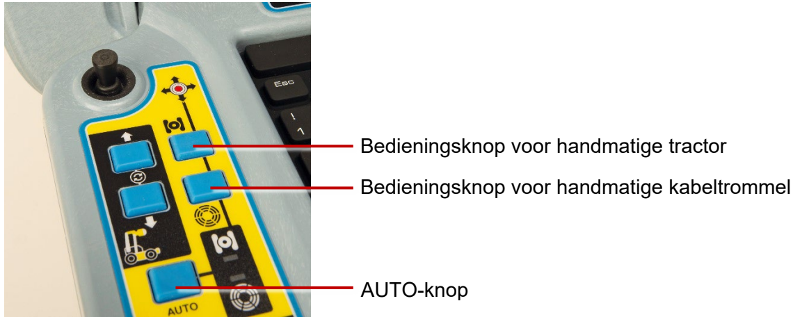
Fig. 6-12 Toetsenbord met AUTO-knop en knoppen voor handmatige tractor en kabeltrommel
