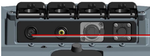
Fig. 4-32: Voedingsbus (1) op het hoofdaansluitingspaneel
